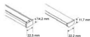
Perfil interm.
