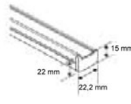
Perfil intermedio
