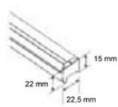
Perfil inferior
