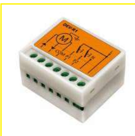
Receptor DEV-R1. Convierte motor mecánico a radio. Sirve también para gestionar Alexa, Google (Siri No) con mando a distancia junto el módulo XDC114S 12E107 (1 x motor o grupo de motores)
